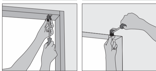
天井付けの場合 正面付けの場合
